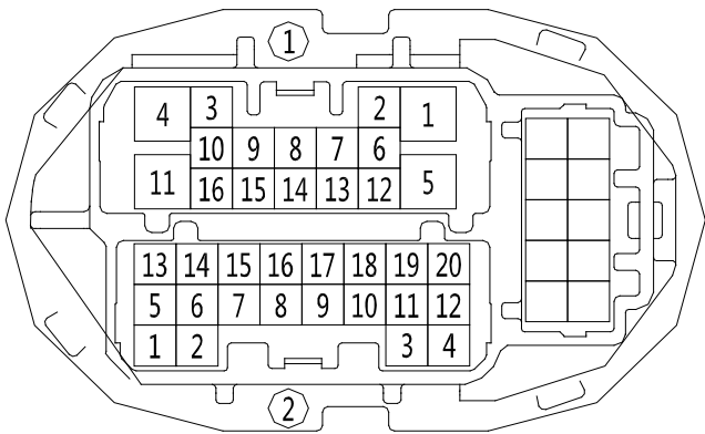
D11--接仪表板线束
