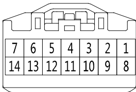
D05--接左前玻璃升降开关
